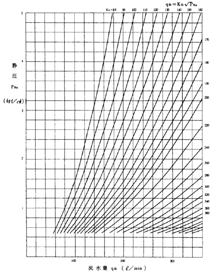
図3-10 流水表
